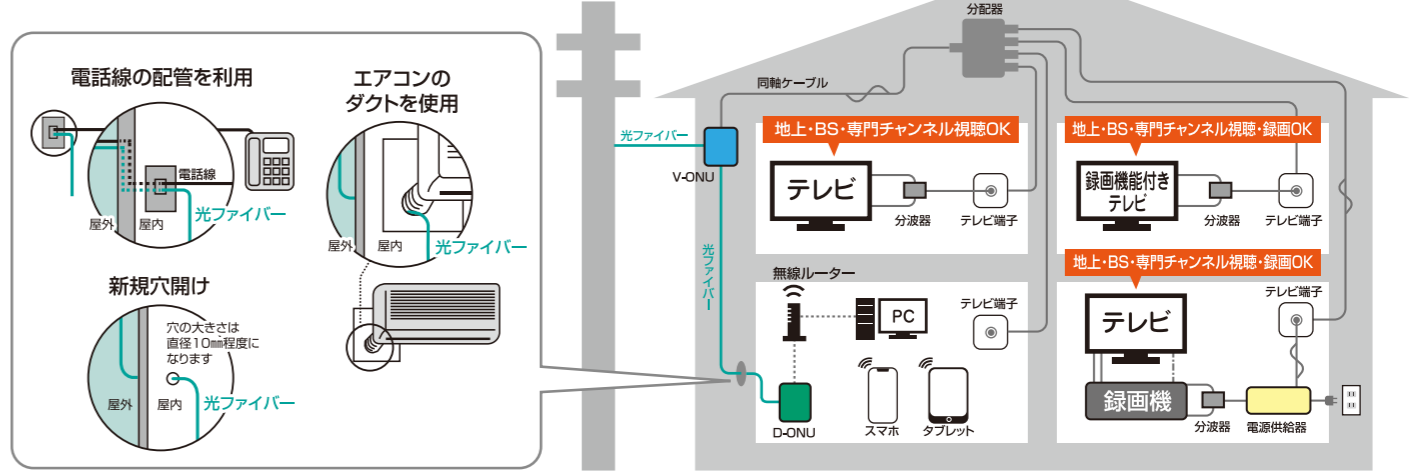
V-ONU:映像用回線終端装置 / D-ONU:通信用光終端装置 ..... LANケーブル / ---- HDMI
